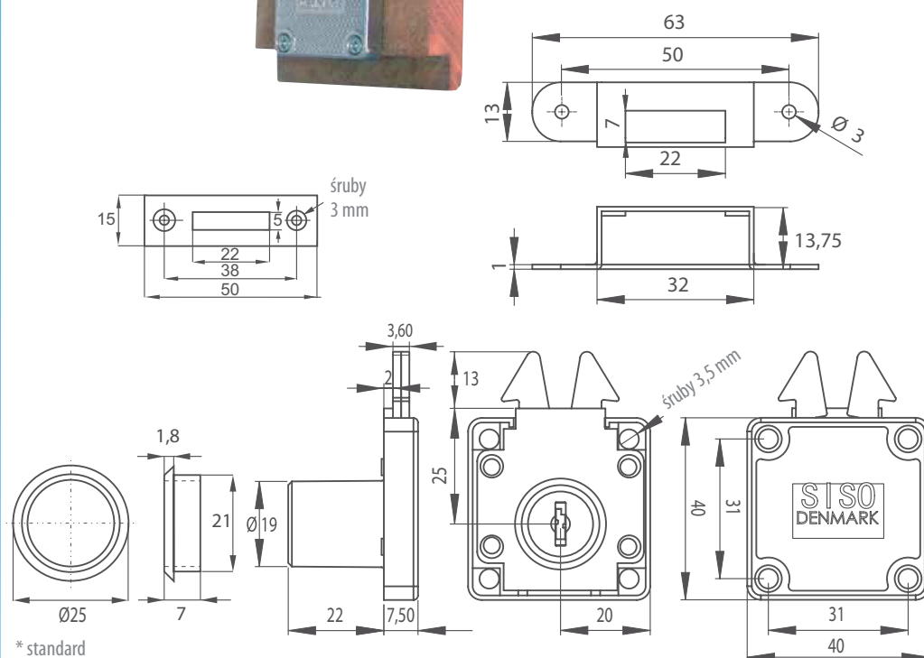
Zamek z wypukłym zaczepem rygla
