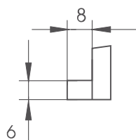
Wymiary klucza
