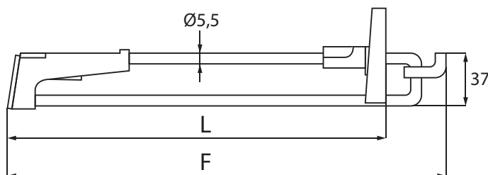
Mocowanie wieszaka w pozycji zamkniętej
