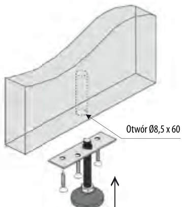
Montaż stopki wspomagającej do płyty
