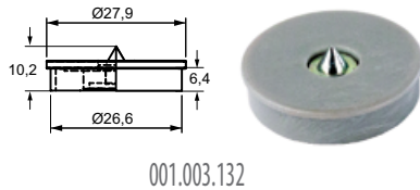
Znacznik
