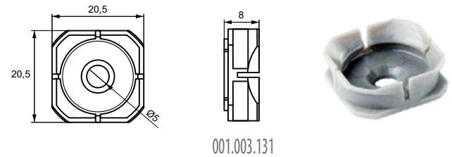
Część żeńska
