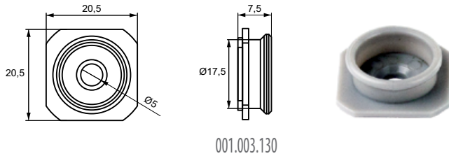
Część męska
