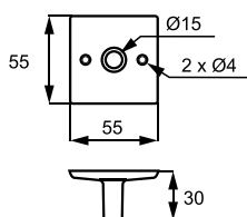
Element łańcucha z łącznikiem
